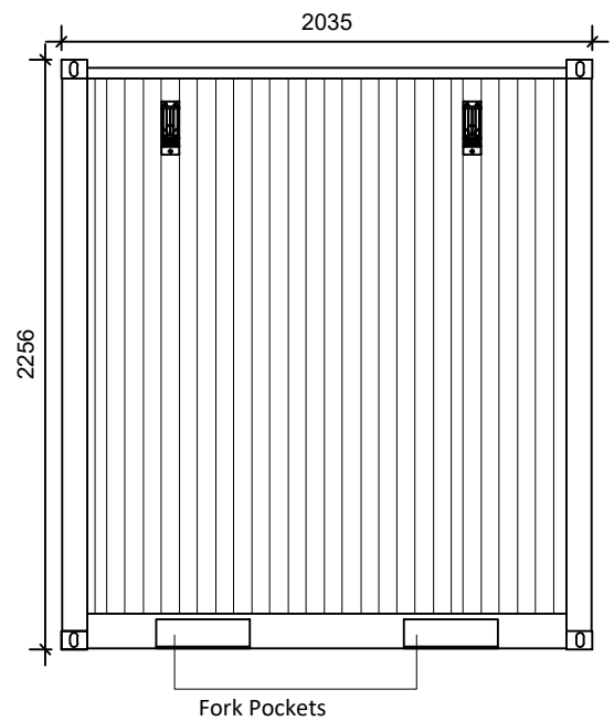
SCALE 1 : 75 MN Container Elev 01
